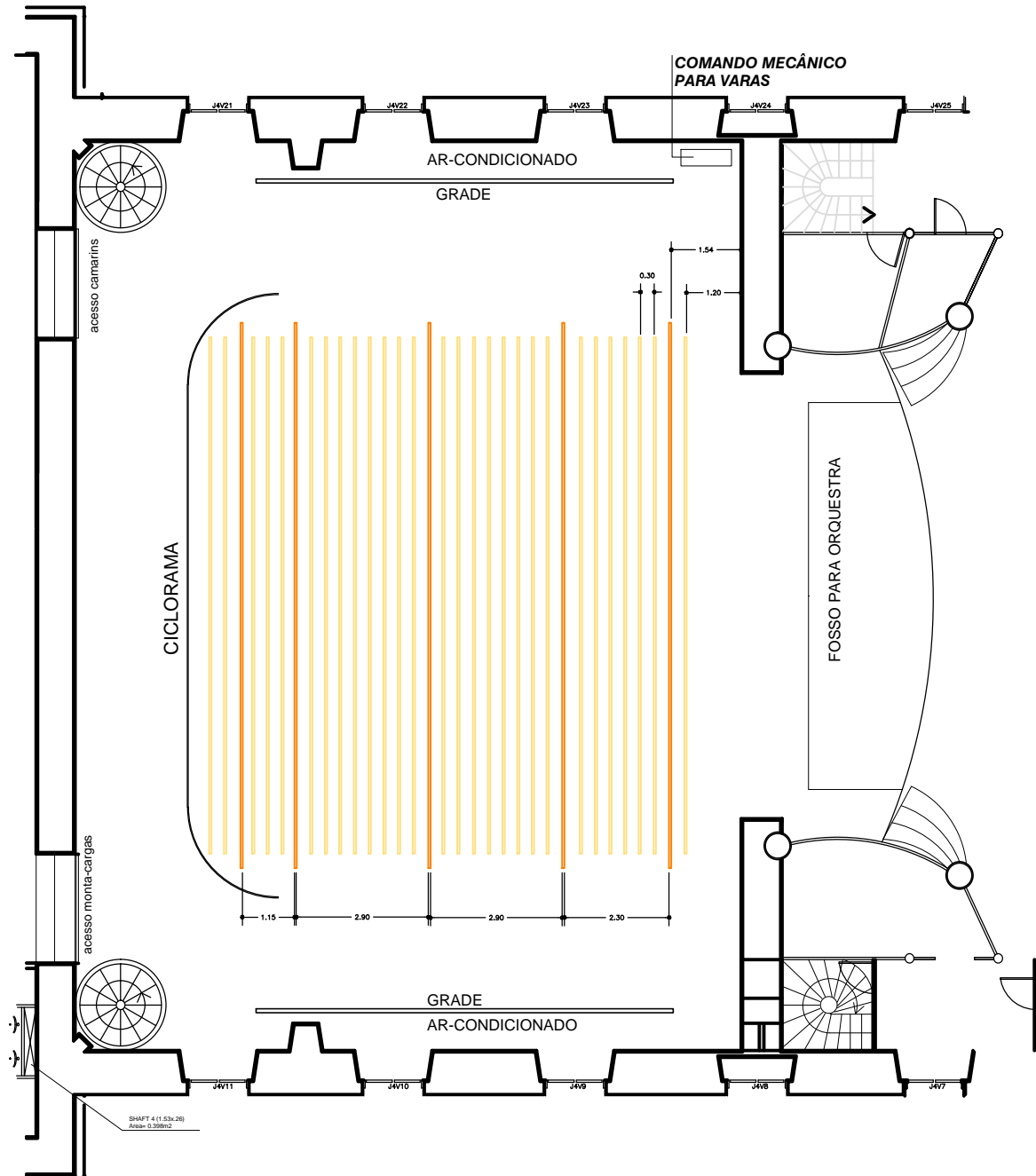
02 PLANTA VARAS DE CENÁRIO E LUZ
